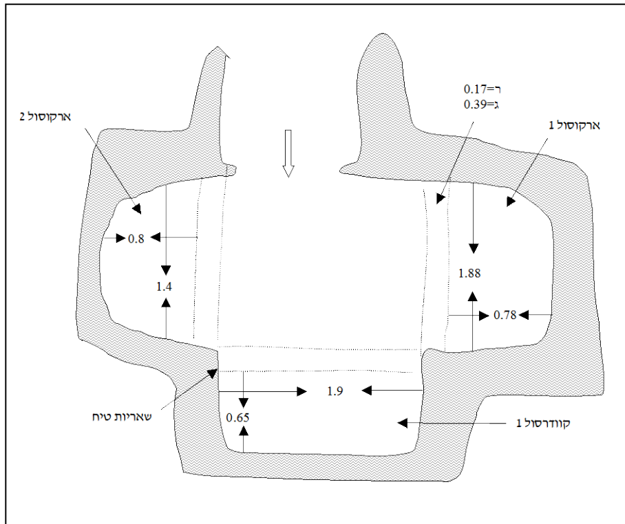
איור מספר 1: סרטוט מערת המנורה.
